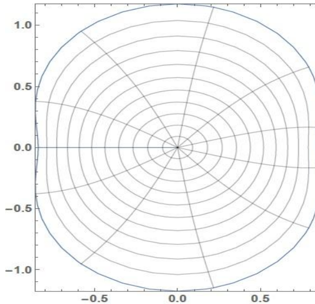
شکل ۱. تصویر قرص واحد تحت تابع \sin z
