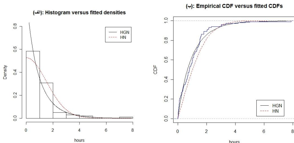
شکل ۶. نمودار تابع چگالی و تابع توزیع مدل‌های برازش داده شده به مجموعه داده تنش-گسیختگی
