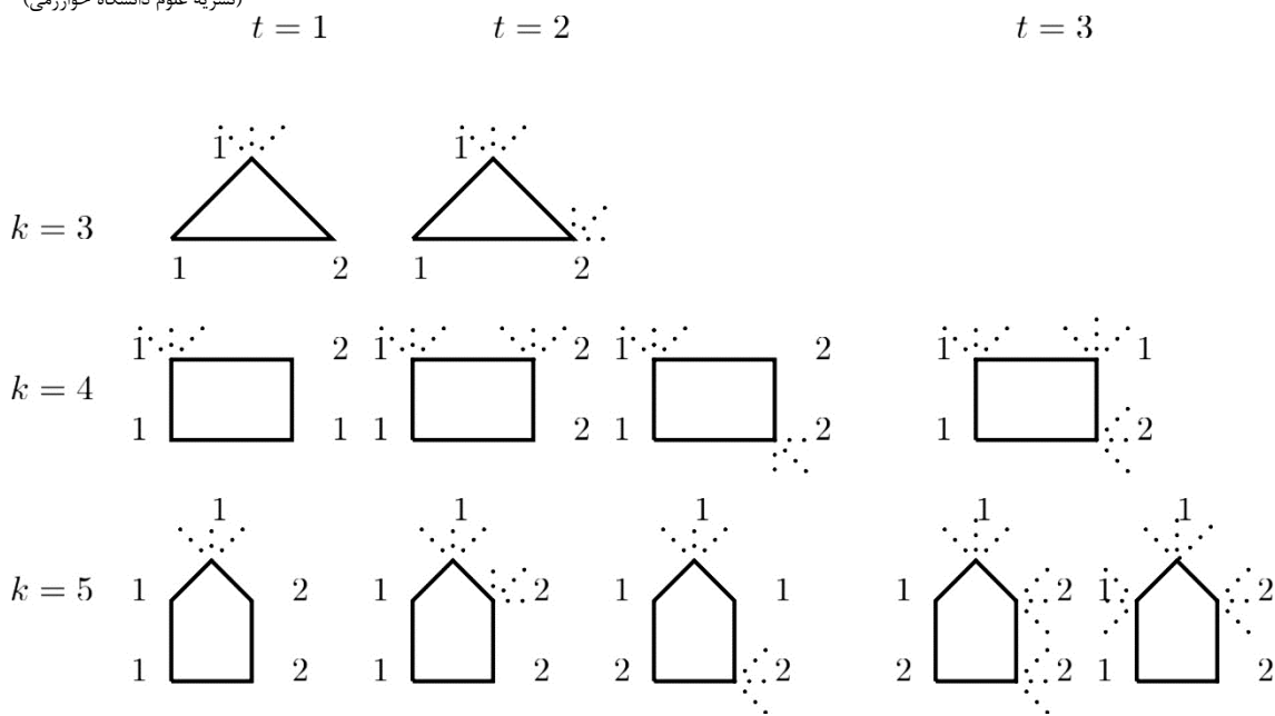
شکل ۳. رنگ آمیزی رئوس دور C در قضیه ۵ حالت ۲۳
