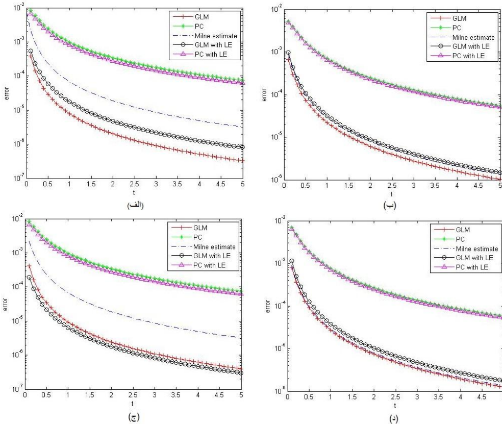
شکل ۲. مقایسه خطاهای روش GLM و PC برای مثال ۷: الف) روش مرتبه دوم حالت PEC، ب) روش مرتبه چهارم حالت (P(EC))^2 ، ج) روش مرتبه دوم حالت (P(EC))^2 ، د) روش مرتبه چهارم حالت (P(EC))^2 . مشابه مثال ۷ این مسله را در بازه زمانی [0,5] با طول گام h = 10^{-2} حل می‌کنیم. تخمین میلن و خطاهای L_\infty برای روش PC مرتبه دوم و چهارم (۳-۶) و (۳-۹) در حالت متناهی PEC و شکل روش خطی کلی آن‌ها (۳-۷) و (۳-۱۰) به ترتیب در جدول ۵ و ۷ ارائه شده‌اند و به‌طور مشابه برای حالت متناهی (P(EC))^2 نتایج عددی در جدول ۶ و ۸ ارائه می‌شوند.
