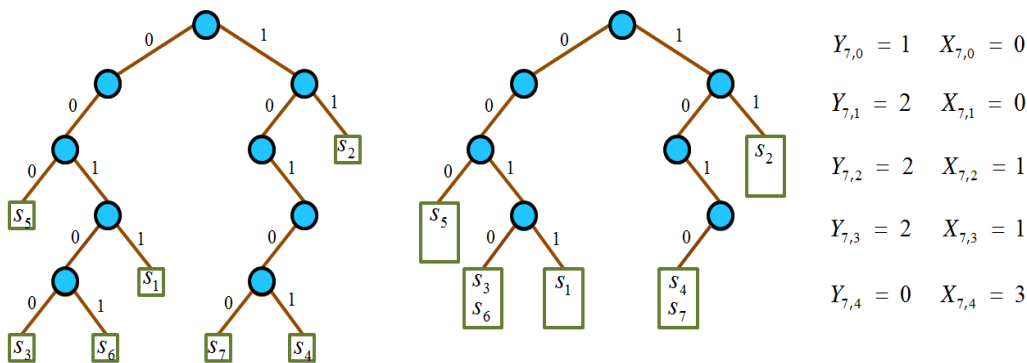
شکل ۱. نمایش یک ترای (درخت سمت چپ) و ترای سطلی (درخت سمت راست) ساخته شده از \mathcal{V} رشته (S_1 = 0011 \dots, S_2 = 11 \dots, S_3 = 0010 \dots) با b = 2 . هم چنین گره‌های داخلی با دایره‌ها (در هر دو ترای)، گره‌های خارجی در ترای با مربع‌ها و در ترای سطلی با مستطیل‌ها (سطل‌ها) نشان داده شده است.
