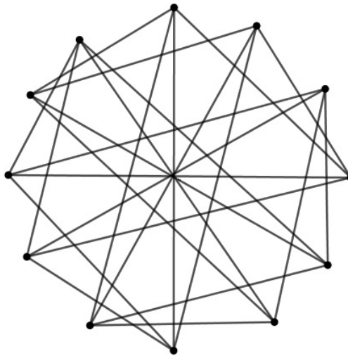
شکل ۳: گراف K_3 \times C_4 .
