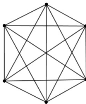
شکل ۱: گراف P_2[K_3] .
