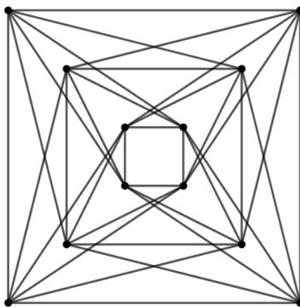
شکل ۵: گراف R_3(G) .
