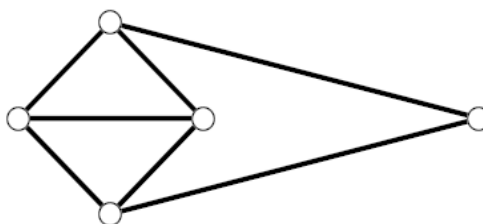
شکل ۳. مثالی از گراف‌ی با خاصیت D(G) < \det(G)
