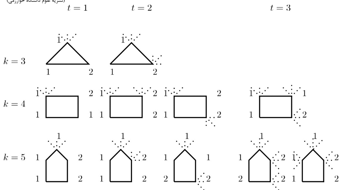
شکل ۳. رنگ‌آمیزی رئوس دور C در قضیه ۵ حالت ۲۳
