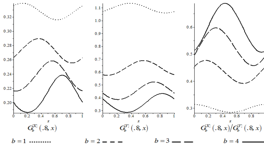
شکل ۲. نمایش منحنی‌های متناوب توابع G_b^{[X]}(.8, x) ، G_b^{[Y]}(.8, x) در یک دوره تناوب، یعنی x \in [0, 1] و
