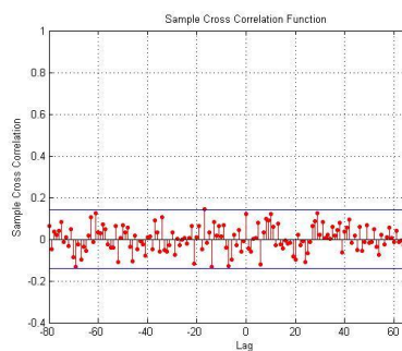
Crosscorr4&amp;5
