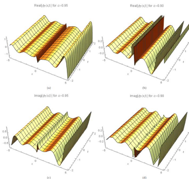
نمودار ۷. شمایل جواب دقیق \phi_7(x,t) ، با استفاده از مقادیر مختلف \alpha و a=0.1, b=0.3, \rho=0.2, \lambda=\theta=\gamma=0.1
