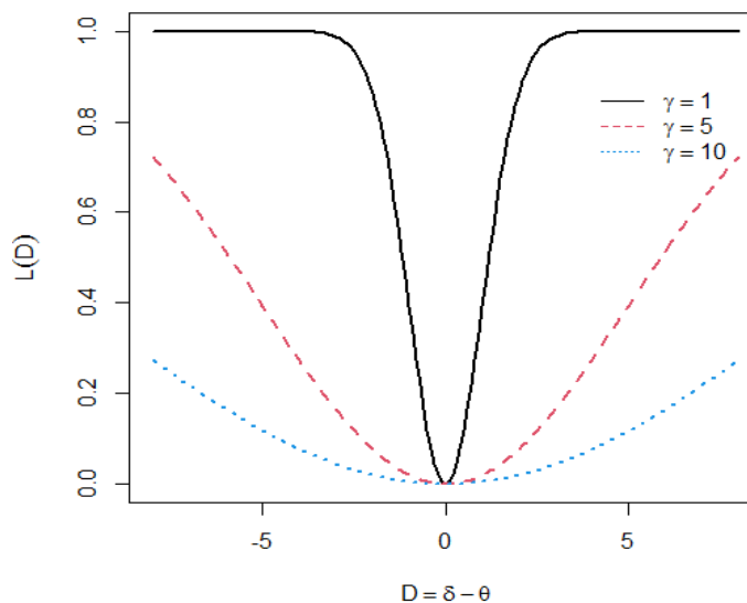
شکل 1: تابع زیان نرمال بازتابیده برای k=1 .
